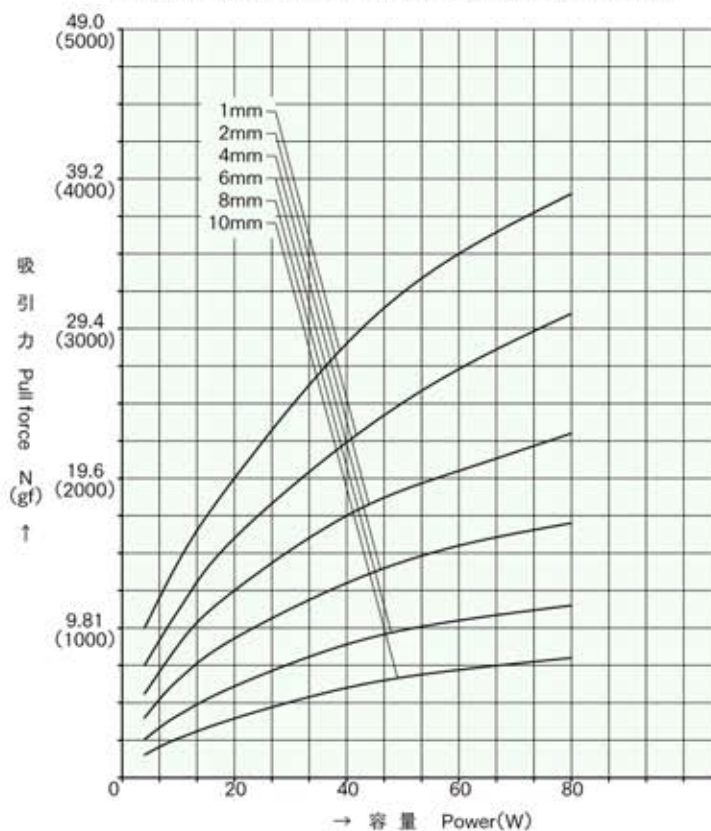
標準コイル表 定格 8W Standard Coil Specifications Rated Power 8W
