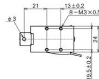
外形寸法 Dimensions
