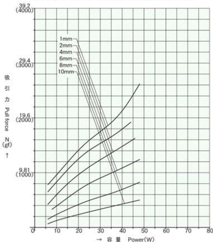
標準コイル表 定格 6W Standard Coil Specifications Rated Power 6W
