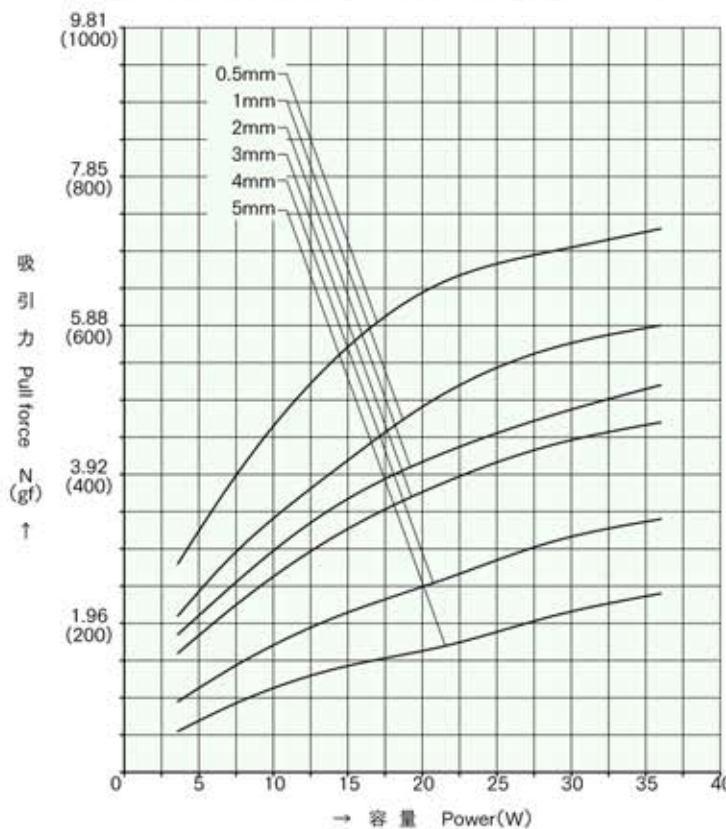
標準コイル表 定格 3.6W Standard Coil Specifications Rated Power 3.6W
