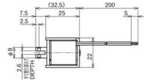
外形寸法 Dimensions
