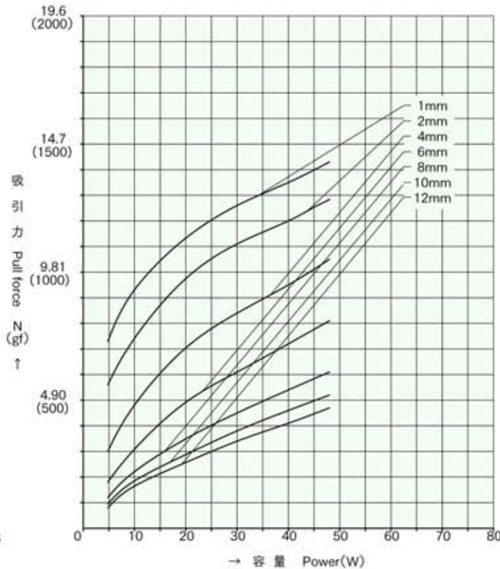
標準コイル表 連続定格 4.8W Standard Coil Specifications Cont. rating 4.8W
