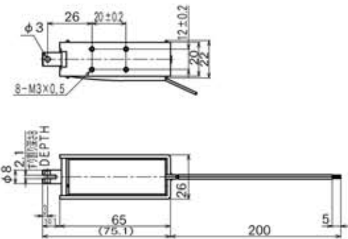
外形寸法 Dimensions
